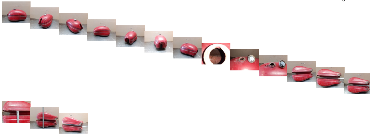
M31-004 image
