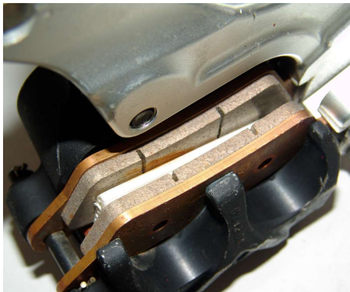
PINZA FRENO POSTERIORE REAR CALIPER BREMBO (BB96)
