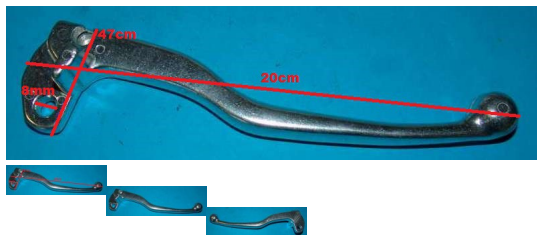
LEVA FRENO SINISTRA PER SCOOTER (LF55)
