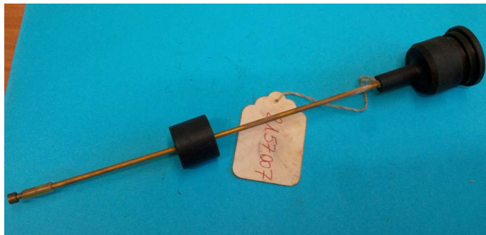
SENSOR FLOAT TANK SENSORE GALLEGGIANTE SERBATOIO
