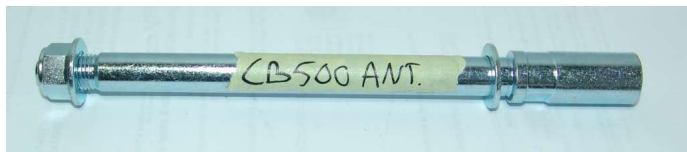
PERNO RUOTA ANTERIORE FRONT AXLE CB 500
