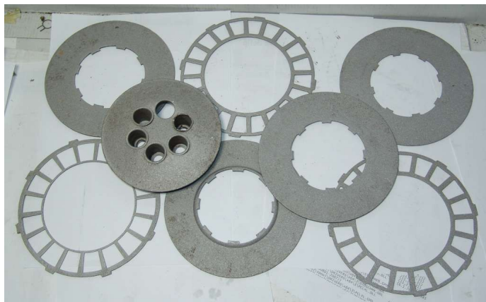
FRIZIONE CLUTCH BIANCHI 500 STELVIO CA969
