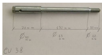
PERNO RUOTA BENELLI MORINI MALANCA CAGIVA DUCATI CV38
