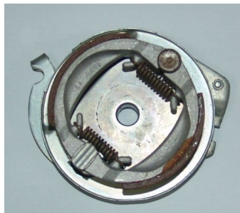
FRENO TAMBURIO PORTA CEPPI GANASCE deluxe Little HONDA 45050-093-001 003 013(4)
