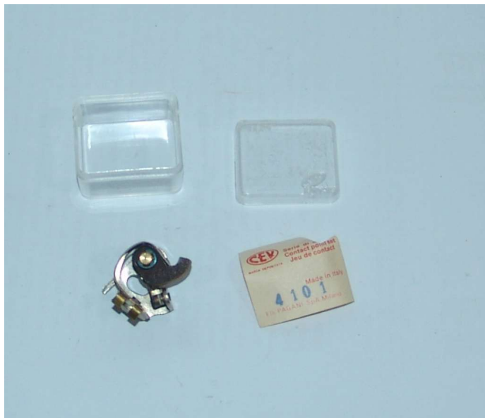
CONTATTI PUNTINE CONTACTS PINS DEMM 125 CEV 4101 TIPO
